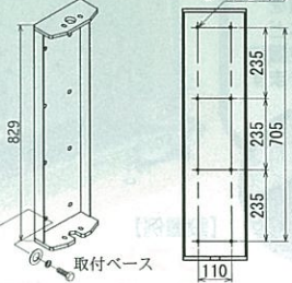
取付ベース寸法図
