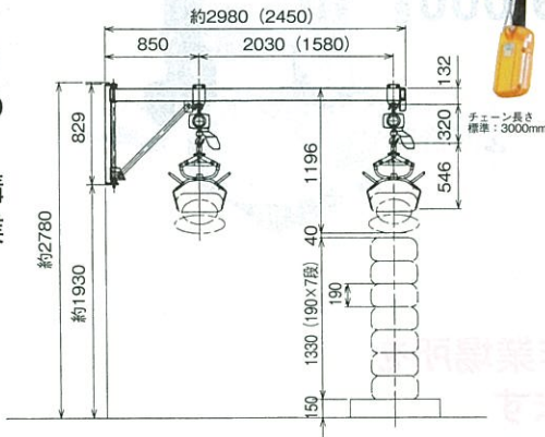
RHL-3000寸法図 ( ) はRHL-2400
