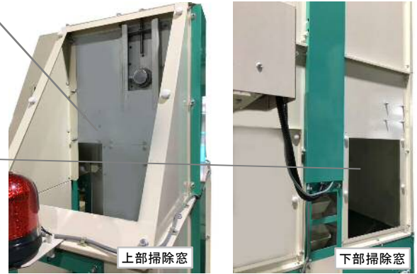
残留米取出
