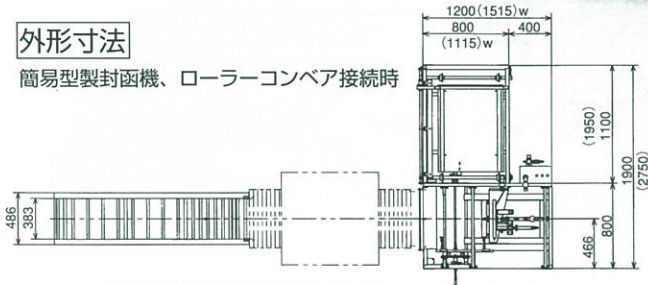
簡易型製封函機
