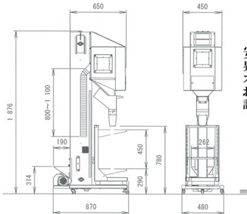
機体寸法(mm)
