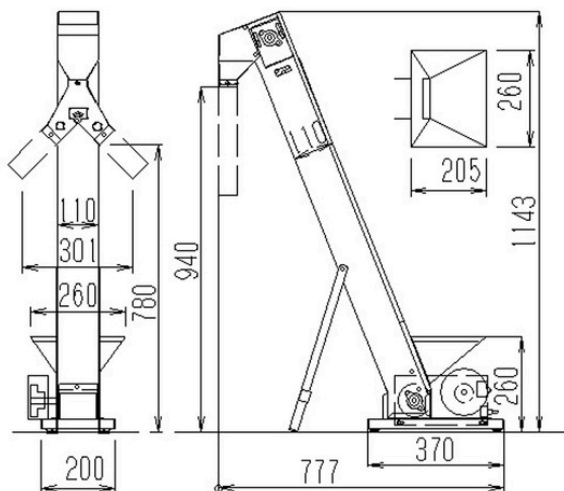
小型昇降機RE9EB外形寸法図
